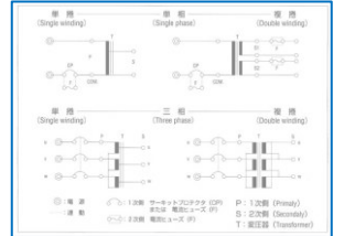
結線図作成
